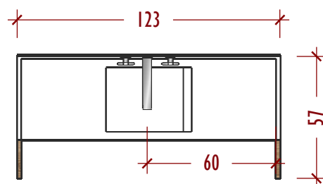
VISTA SUPERIOR
