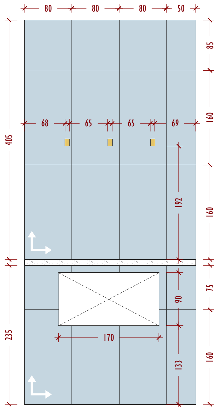
PAGINAÇÃO PAREDE
