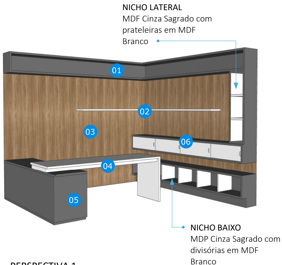
PERSPECTIVA 1
