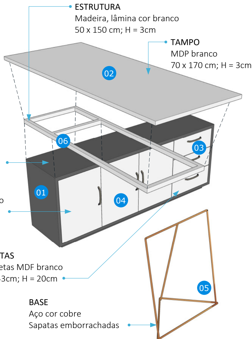
PERSPECTIVA EXPLODIDA
