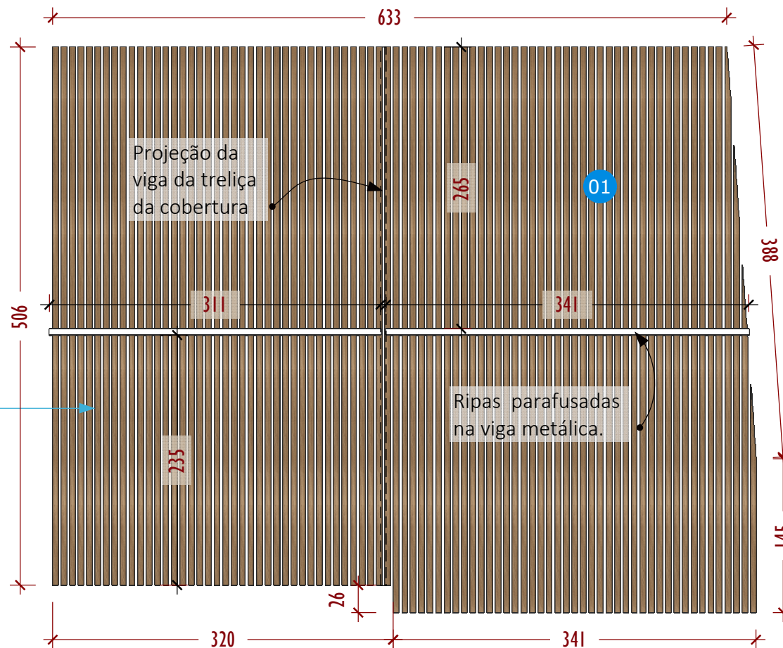
VISTA SUPERIOR - SEÇÃO 2
