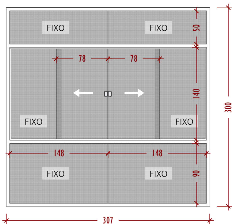
ESQUADRIA 03
