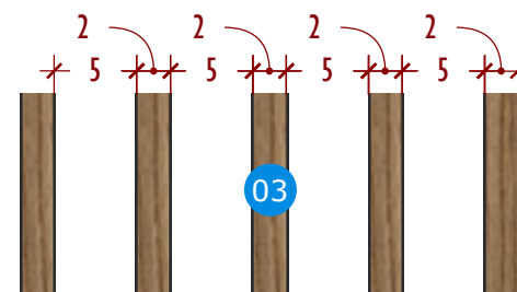
DETALHE RIPADO ESC. - 1 : 5
