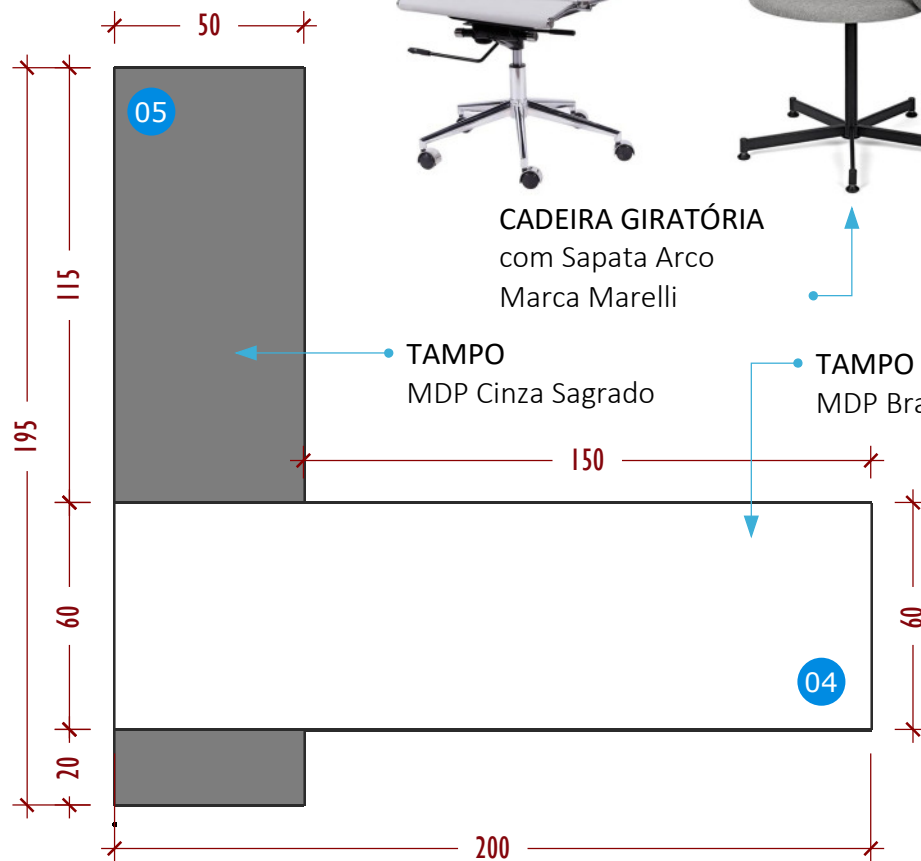
VISTA SUPERIOR
