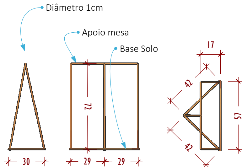
VISTAS DA BASE
