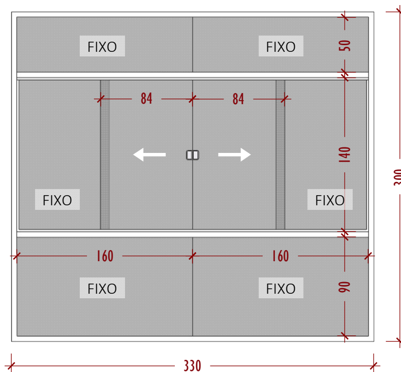
ESQUADRIA 02
