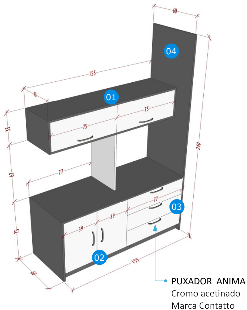
PERSPECTIVA 1
