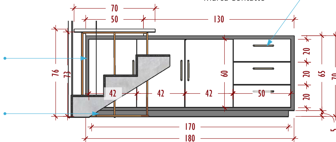
VISTA LATERAL
