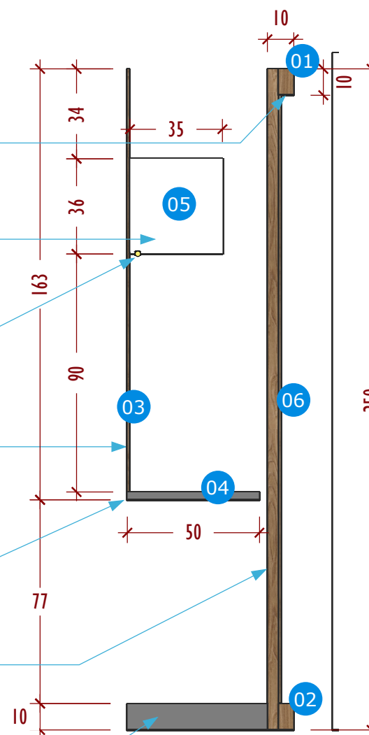
VISTA LATERAL
