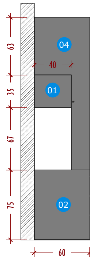
VISTA LATERAL
