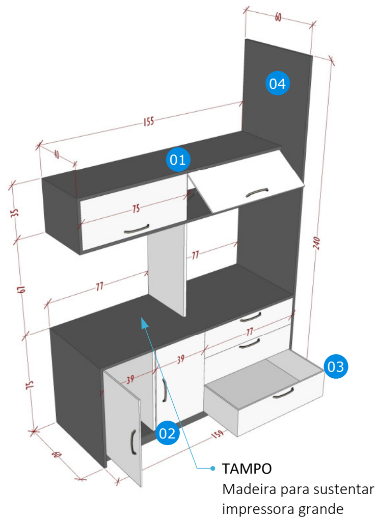
PERSPECTIVA 2
