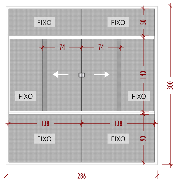
ESQUADRIA 01
