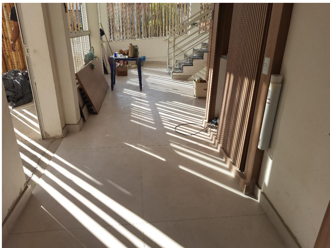
Figura 7 – Aplicação de porcelanato e rodapé no 1º Pavimento.
