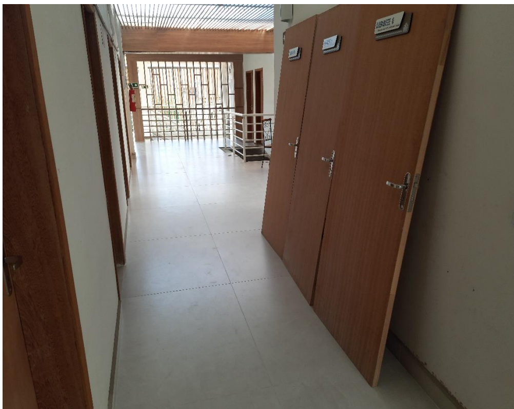
Figura 29 – Aplicação de porcelanato e rodapé no 2º Pavimento.
