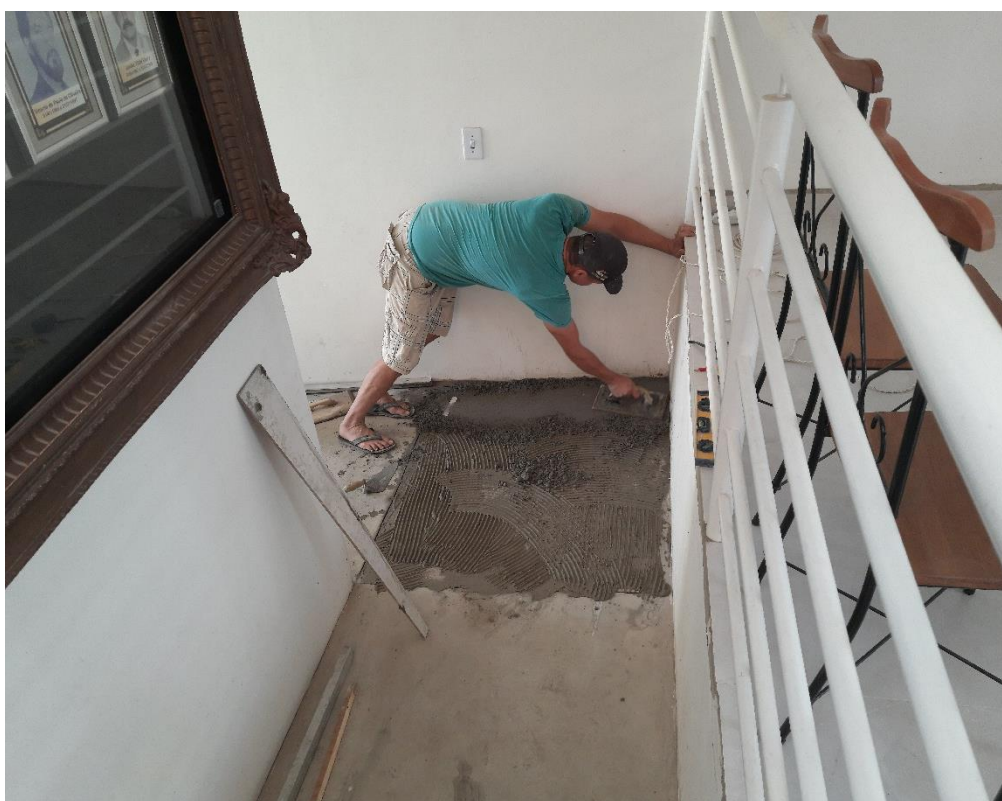
Figura 41 – Aplicação de porcelanato e rodapé no 2º Pavimento. Execução de contra-piso.
